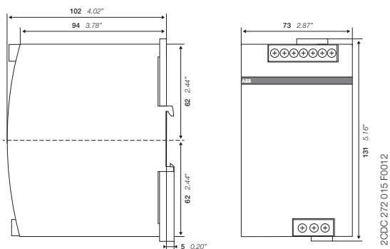
CP-ASI 4.0
