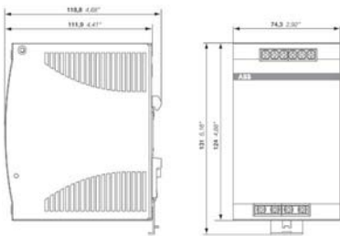
CP-T 24/5.0
